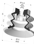
Sauggreifer 2.5 Falten Serie 96C Ø 30MM Produktreferenz: 96C 30-- A
