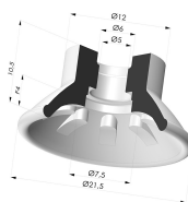
Flachsauggreifer Serie 99 Ø 21.5 mm
