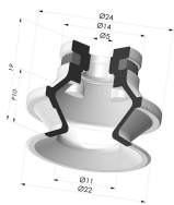
Sauggreifer 1.5 Falten Serie 91 Ø 22,2MM
