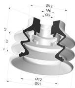
Sauggreifer 2.5 Falten Serie 96C Ø 20MM
