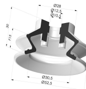
Sauggreifer 1.5 Falten Serie 97B Ø 52.5MM
