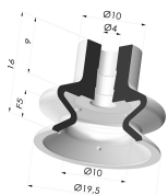
Sauggreifer 1.5 Falten Serie 1 Ø 20MM -mit Auslöser Produktreferenz: 1 20--A SPD
