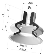
Sauggreifer 1.5 Falten Serie 1 Ø 23MM - mit Auslöser Produktreferenz: 1 23--A SPD
