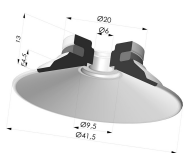
Flachsauggreifer Serie 9 Ø 41,5MM
