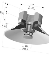
Flachsauggreifer Serie 9 Ø 41.5MM
