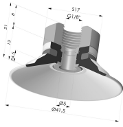
Flachsauggreifer Serie 9 Ø 41.5MM
