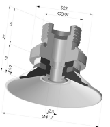
Flachsauggreifer Serie 9 Ø 41.5MM
