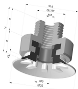
Flachsauggreifer Serie 90 Ø 22MM
