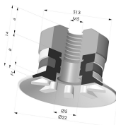
Flachsauggreifer Serie 9 Ø 22MM
