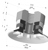
Flachsauggreifer Serie 9 Ø 22MM
