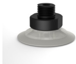
Variantenreferenz: 90 30TPU M18 • Farbe: Transluzent • Materiale: Thermoplastisch • Shore-Härte: SH70
