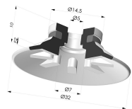
Flachsauggreifer Serie 90 Ø 31,8MM Produktreferenz: 90 30-- A
