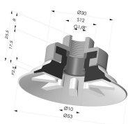
Flachsauggreifer Serie 90 Ø 53MM
