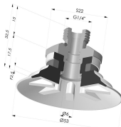
Flachsauggreifer Serie 9 Ø 53MM
