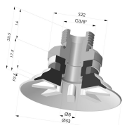
Flachsauggreifer Serie 9 Ø 53MM
