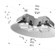
Flachsauggreifer Serie 90 Ø 75MM
