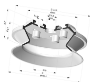
Sauggreifer 1.5 Falten Serie 91 Ø 159,5MM
