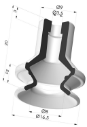
Sauggreifer 1.5 Falten Serie 91 Ø 16,5MM
