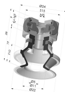
Sauggreifer 1.5 Falten Serie 91 Ø 22.2MM
