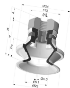
Sauggreifer 1.5 Falten Serie 91 Ø 22.2MM
