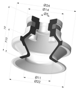
Sauggreifer 1.5 Falten Serie 91 Ø 22,2MM Produktreferenz: 91 20-- A
