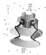
Sauggreifer 1.5 Falten Serie 91 Ø 34MM
