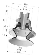
Sauggreifer 1.5 Falten Serie 91 Ø 34MM
