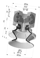
Sauggreifer 1.5 Falten Serie 91 Ø 34MM
