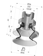
Sauggreifer 1.5 Falten Serie 91 Ø 34MM
