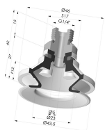
Sauggreifer 1.5 Falten Serie 91 Ø 40MM
