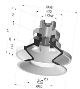
Sauggreifer 1.5 Falten Serie 91 Ø 50MM
