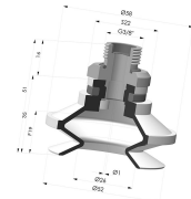
Sauggreifer 1.5 Falten Serie 91 Ø 50MM
