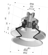
Sauggreifer 1.5 Falten Serie 91 Ø 50MM
