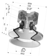
Sauggreifer 1.5 Falten Serie 91 Ø 50MM
