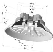
Flachsauggreifer Serie 94 Ø 100MM
