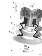
Sauggreifer 2.5 Falten Serie 96 Ø 25MM
