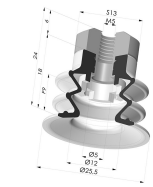
Sauggreifer 2.5 Falten Serie 96 Ø 25MM
