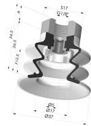
Sauggreifer 2.5 Falten Serie 96 Ø 35MM
