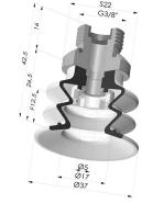
Sauggreifer 2.5 Falten Serie 96 Ø 35MM
