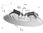
Flachsauggreifer Serie PFG Ø 198 mm
