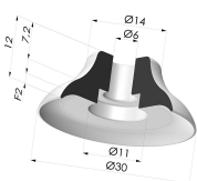
Flachsauggreifer Serie PFG Ø 30 mm
