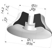
Flachsauggreifer Serie PFG Ø 36 mm
