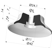
Flachsauggreifer Serie PFG Ø 42 mm Produktreferenz: PFG 40-- A
