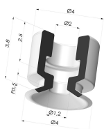
Flachsauggreifer PFG Ø 4 mm
