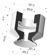
Flachsauggreifer Serie PFG Ø 5.3 mm
