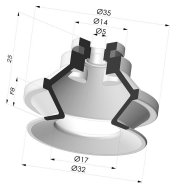
Sauggreifer 1.5 Falten Serie 91 Ø 31,8MM
