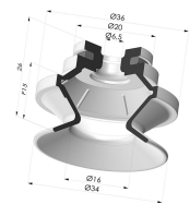
Sauggreifer 1.5 Falten Serie 91 Ø 34MM Produktreferenz: 91 31-- A
