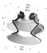
Sauggreifer 1.5 Falten Serie 91 Ø 34MM
