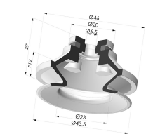
Sauggreifer 1.5 Falten Serie 91 Ø 40MM Produktreferenz: 91 40-- A
