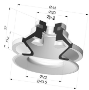
Sauggreifer 1.5 Falten Serie 91 Ø 40MM
