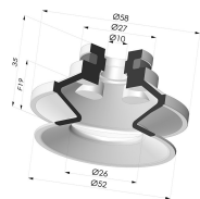
Sauggreifer 1.5 Falten Serie 91 Ø 50MM Produktreferenz: 91 50-- A
