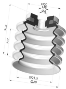
Sauggreifer 4.5 Falten Serie 92 Ø 30MM
