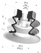
Sauggreifer 2.5 Falten Serie 96 Ø 25MM
