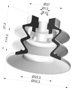
Sauggreifer 2.5 Falten Serie 96 Ø 52MM
