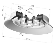
Flachsauggreifer Serie PFG Ø 116.5 mm
