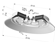
Flachsauggreifer Serie PFG Ø 198 mm
