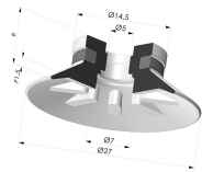
Ventosa Plana Serie 90 Ø 27MM Referencia del producto: 90 25-- A
