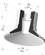
Ventosa Plana Serie 9 Ø 16MM
