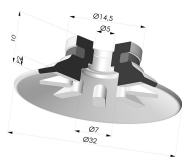
Ventosa Plana Serie 90 Ø 31,8MM
