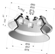
Ventosa 1.5 Fuelles Serie 91 Ø 75MM
