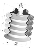
Ventosa 4.5 Fuelles Serie 92 Ø 50MM
