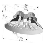
Ventosa Plana Serie 94 Ø 100MM
