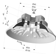
Ventosa Plana Serie 94 Ø 100MM
