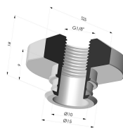
Conexión Desmontable Hembra 1/8G
