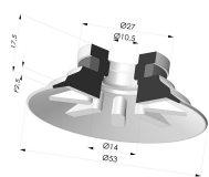
Ventosa Plana Serie 90 Ø 53MM
