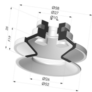
Ventosa 1.5 Fuelles Serie 91 Ø 50MM Referencia del producto: 91 50-- A
