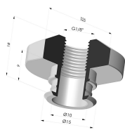
Conexión Desmontable Hembra 1/8G Referencia del producto: 9G18-2
