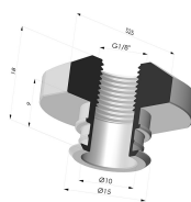
Conexión Desmontable Hembra 1/8G
